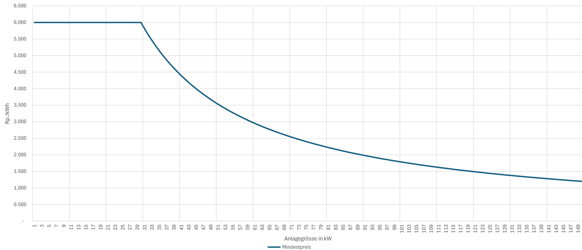
Mindestpreis für Rückvergütungen für PV-Anlagengrößen von 30 kW bis 150 kW mit Eigenverbrauch
